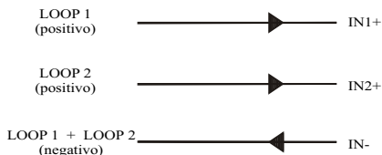
FIG. 6 LOOP 4...20 mA (alimentato)
