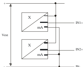
FIG. 5 TRASMETTITORI 4...20 mA 3 fili ALIMENTATI ESTERNAMENTE (Vext)
