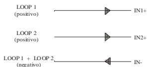
FIG. 6 LOOP 4...20 mA (alimentato)
