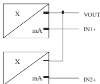
FIG. 3 TRASMETTITORI 4...20 mA 2 fili ALIMENTATI DAL DISPOSITIVO
