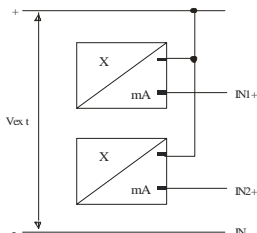
FIG. 4 TRASMETTITORI 4...20 mA 2 fili ALIMENTATI ESTERNAMENTE (Vext)
