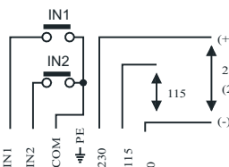
INGRESSI DIGITALI
